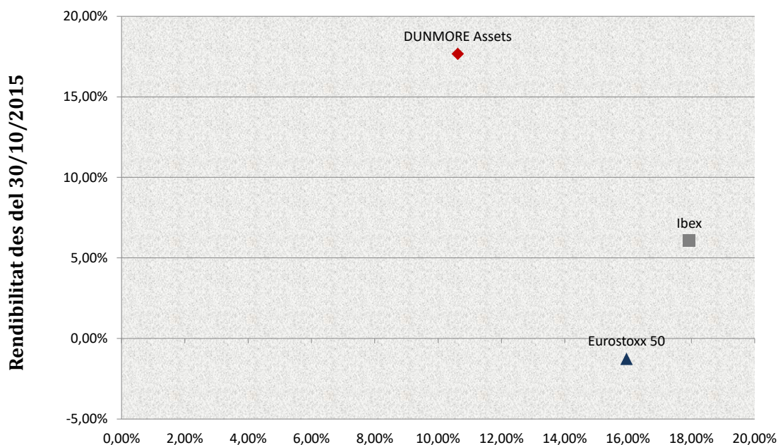
Volatilitats anualitzades
